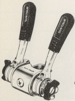
UB-10 No. 3030
